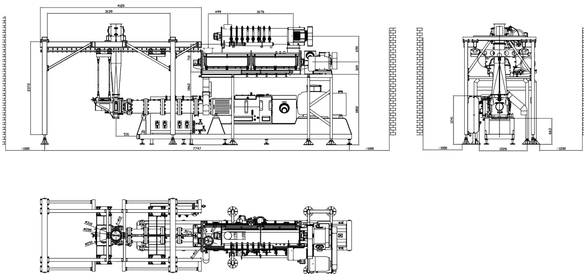
Desenho Técnico da SPHS 100 x 2
